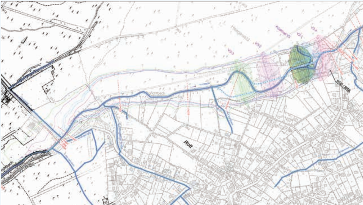
Lagepläne der Varianten für die Hochwasserrück- haltebecken an der Vicht
