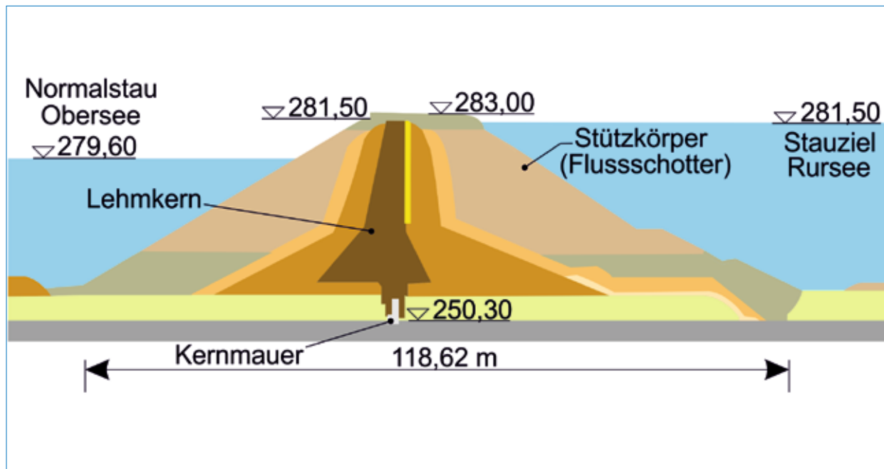
Detail aus dem Regelquerschnitt des Bestandplans des Paulushofdammes
