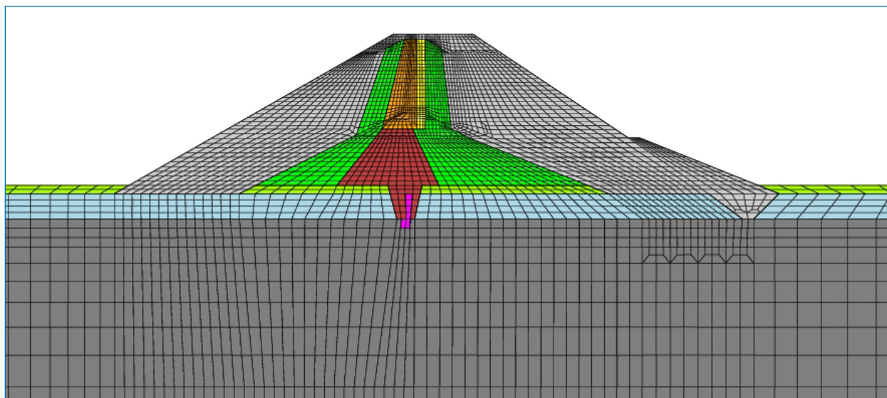
Detail aus dem Regelquerschnitt Finite-Elemente-Modell des Paulushofdammes im Rahmen der Standsicherheitsüberprüfung
